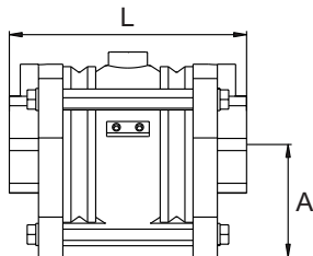
דגם 711 מתוברג
